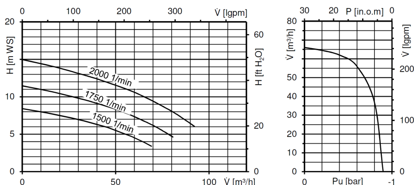
Pumpenkennlinie 2000 1/min, berechnete Werte für 1750 1/min und 1500 1/min: Bezug: p u = 0 bar Unterdruck
